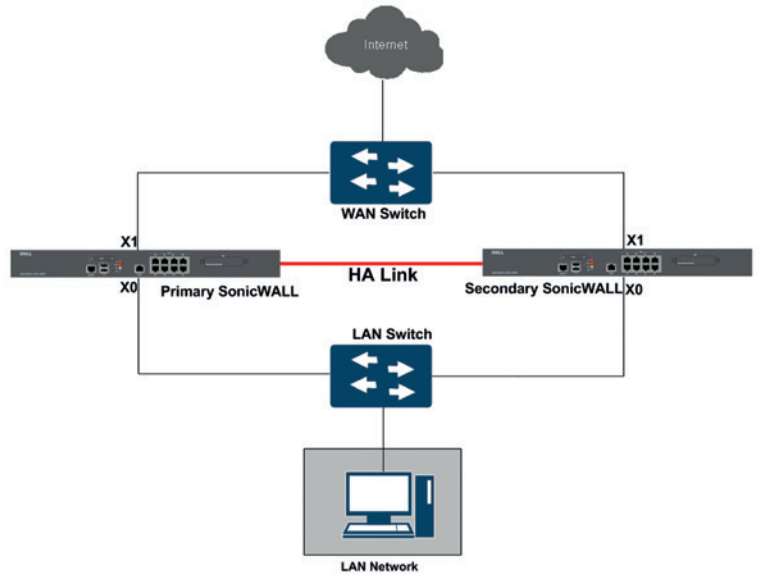
Obr.: Schéma zapojení firewallů Dell SonicWall v režimu HA
